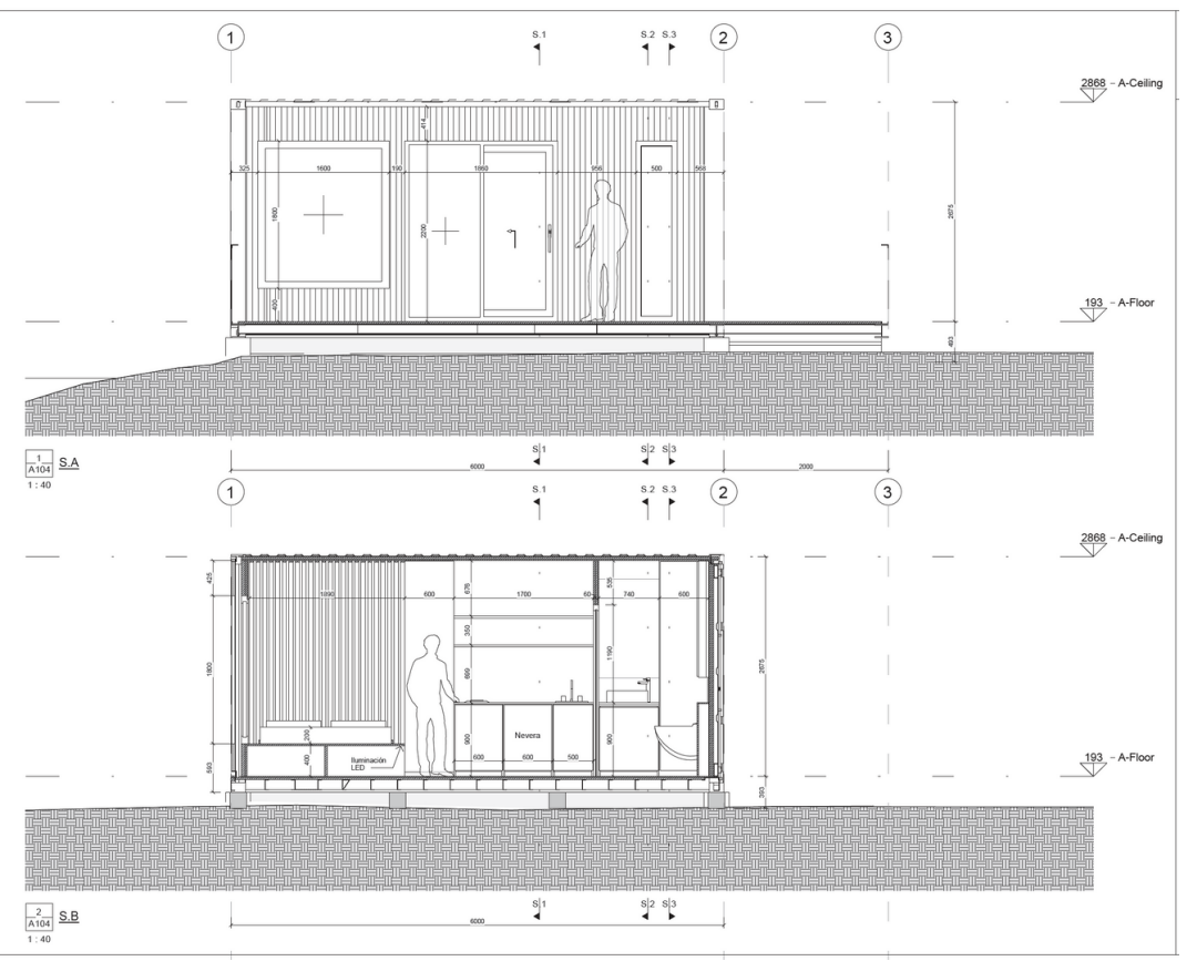
Propuesta diseño_#001
